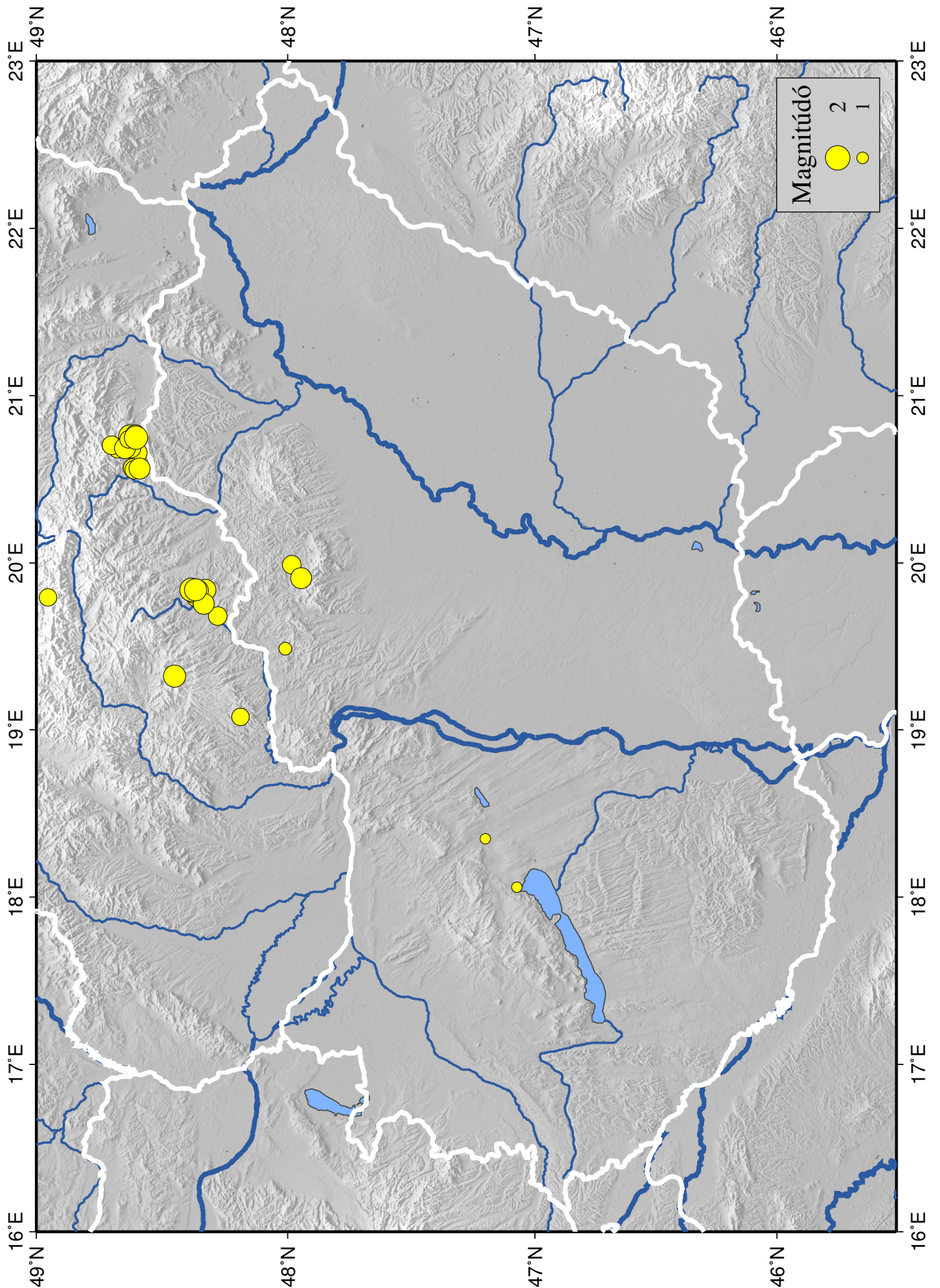
1.3. ábra. A 2013-as év azonosított és valószínűsíthető robbantásainak epicentrumai
